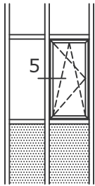
CEPHE İÇERİSİNE EW 55 SİSTEM İÇE AÇILIR GİZLİ KANAT DETAYI
