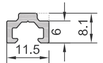
K 894 | Yükseltme Çıtası Pr. 0,110 kg/m | Spacer Pr. Profil no:10122
