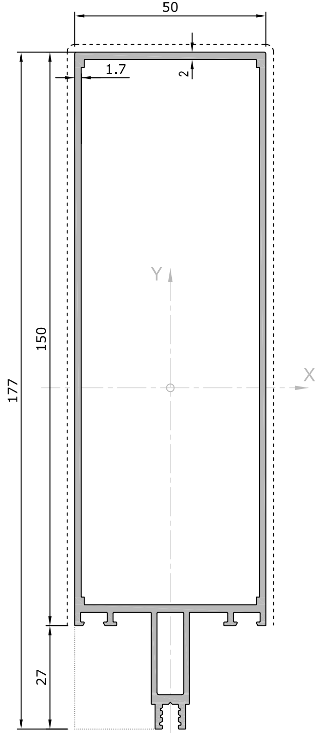
8014 | 150 'lık Düşey ve Yatay 2,255 kg/m Mullion and Transom Profile Jx=278,19 cm 4 | Jy=33,99 cm 4
