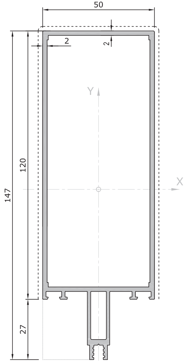
8032* | 120 'lık Düşey ve Yatay 2,150 kg/m | Mullion and Transom Profile J_x=174,84 \text{ cm}^4 | J_y=31,52 \text{ cm}^4
