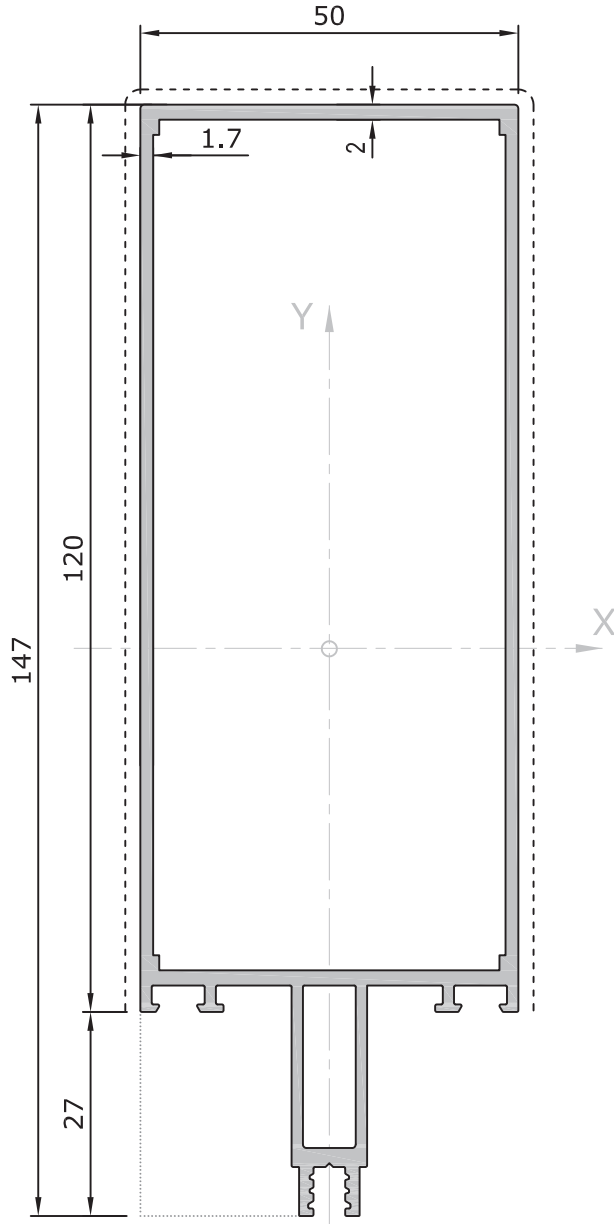
8013 | 120 'lık Düşey ve Yatay 1,980 kg/m | Mullion and Transom Profile J_x=167,32 \text{ cm}^4 | J_y=28,03 \text{ cm}^4
