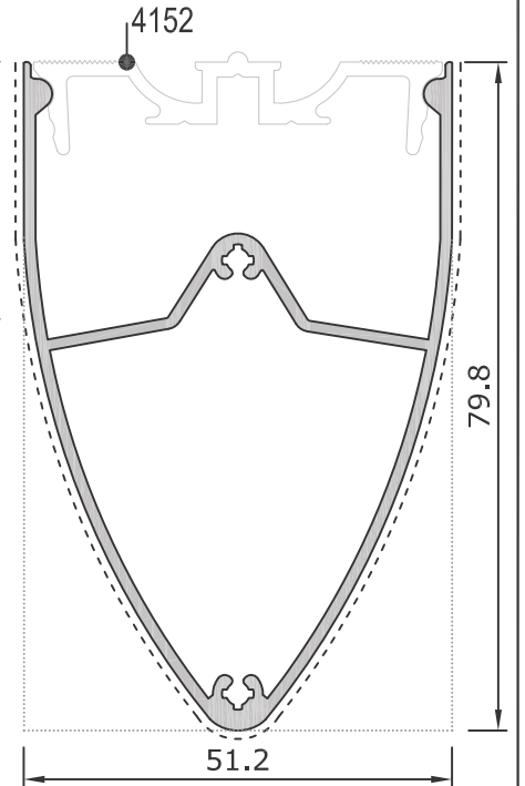
283 | 80 mm Badem Kapak Profili Pr. 1,045 kg/m Cover Cap Pr.
