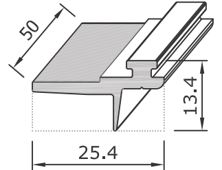
8084 | Cam Altı Destek Pr. 0,245 kg/m | Glazing Support Pr. Mat Siyah Elokso / Matte Black Anodized
