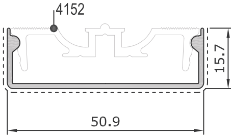
4153-D | 15,7 mm Kapak Profili Pr. 0,310 kg/m Cover Cap Pr.
