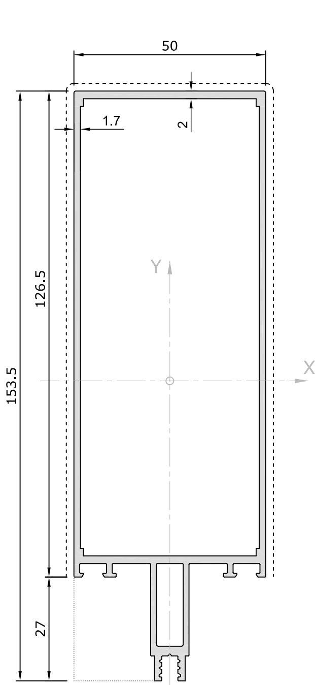
8085* | 126,5 'lık Düşey ve Yatay 2,035 kg/m | Mullion and Transom Profile Jx=188,42 cm 4 | Jy=29,32 cm 4
